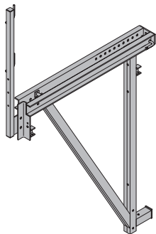
悬挂托架 D15/3 Sperrkonsole D15/3
