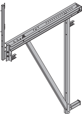
悬挂托架 D22 K Sperrkonsole D22 K
