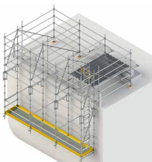
Ponteggio sospeso
